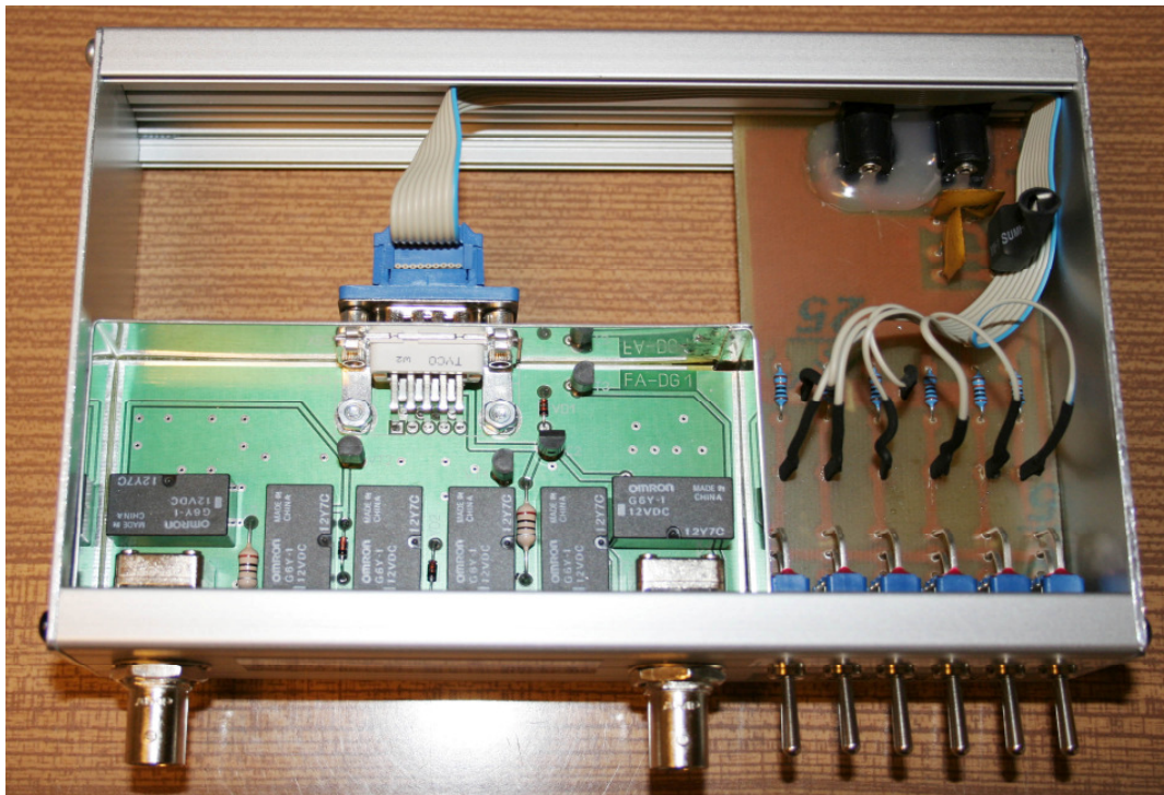
FA-NWT Dämpfungsglied:
